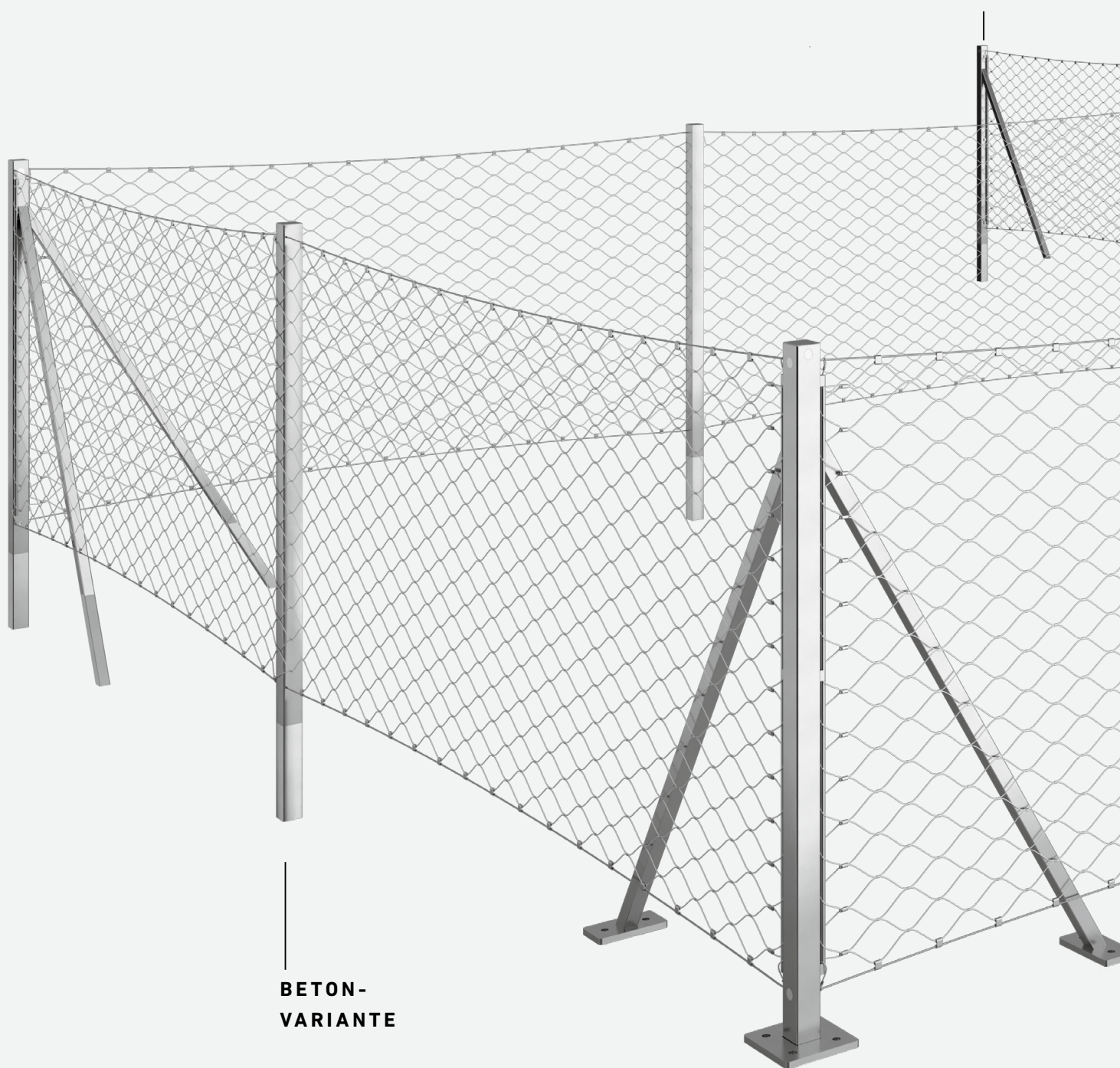
END- PFOSTEN
